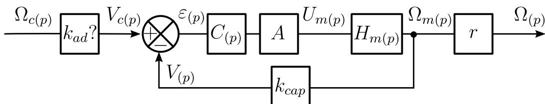
FIGURE 2 – Schéma-bloc — asservissement de vitesse
